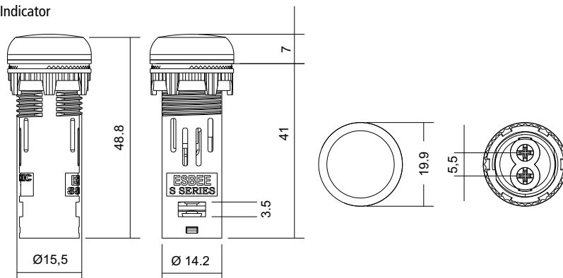
16 mm Indicator
